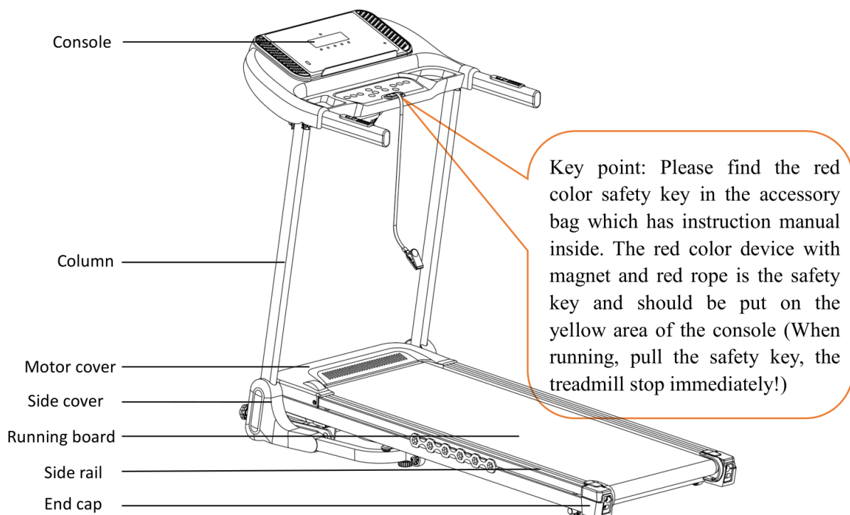
Основні компоненти бігової доріжки
